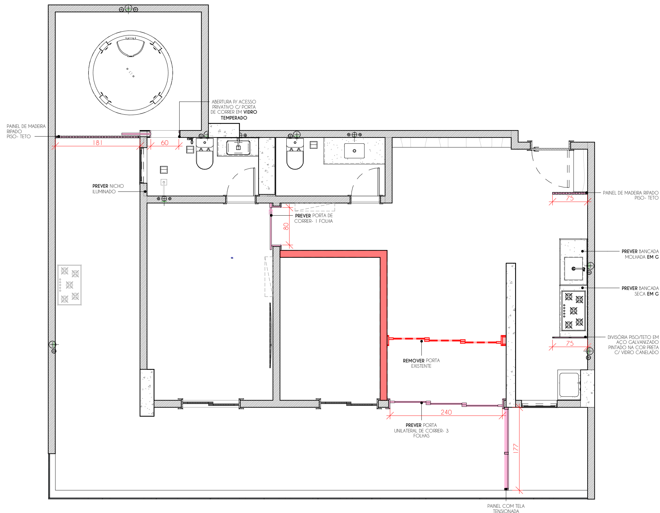
PLANTA BAIXA- DEMOLIÇÃO E CONSTRUÇÃO ESCALA 1 : 50
