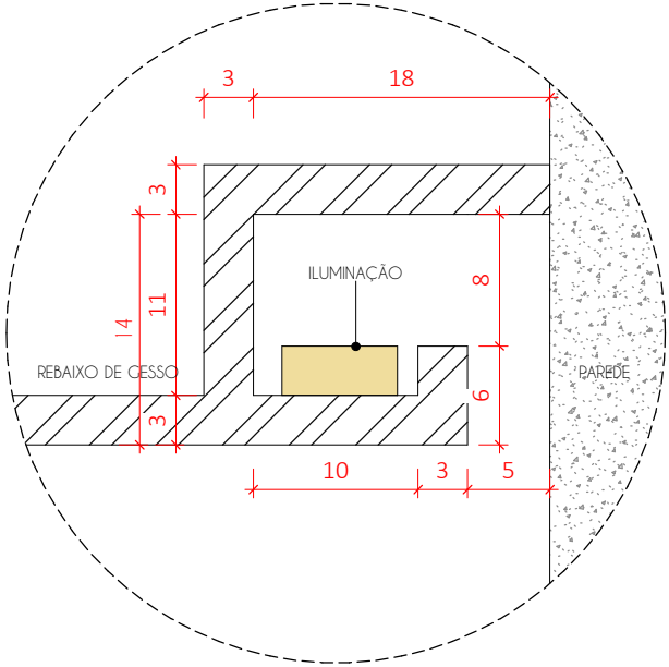
DET. LINHA DE SOMBRA ESCALA 1 : 5
