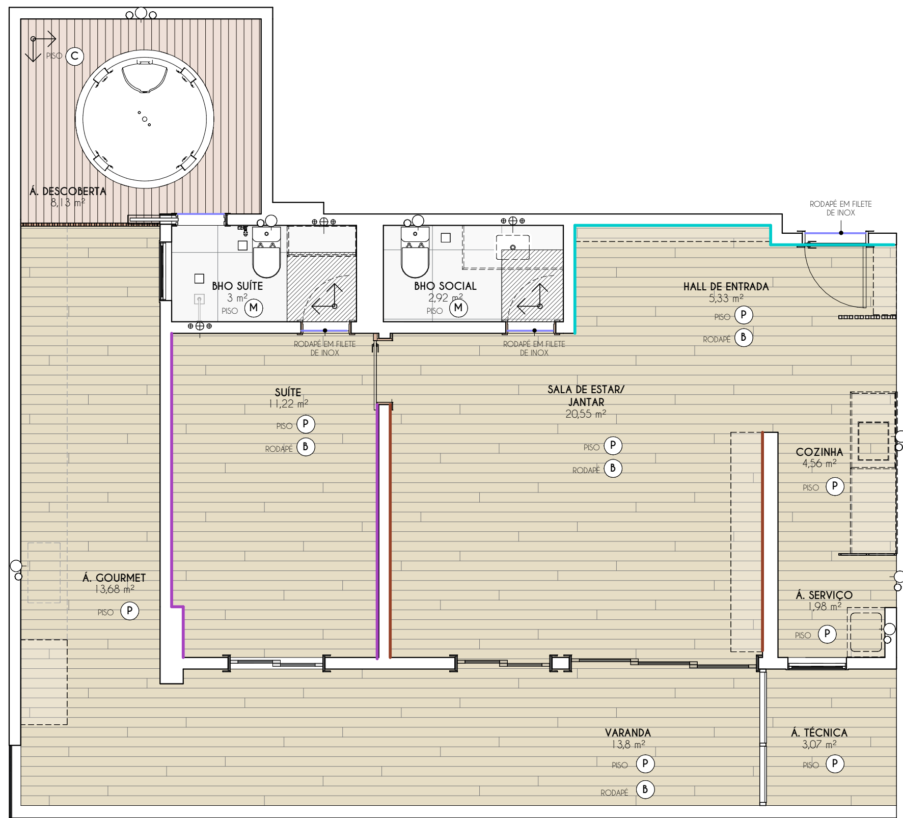
PLANTA BAIXA- PAG. PISO E ACABAMENTOS ESCALA 1 : 50
