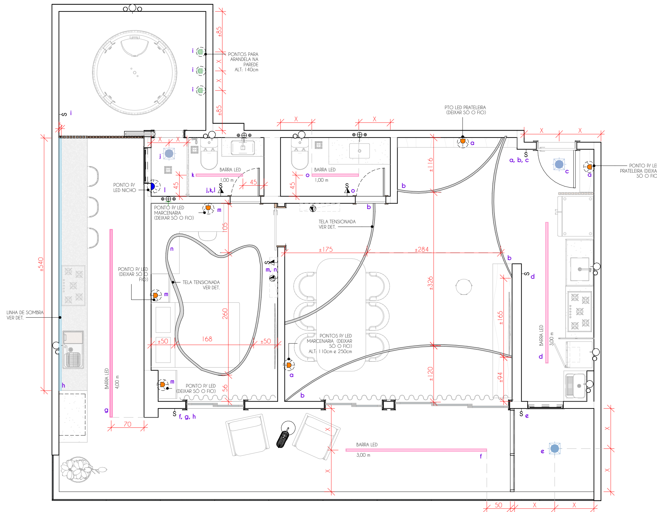
PLANTA BAIXA- ILUMINAÇÃO ESCALA 1 : 50
