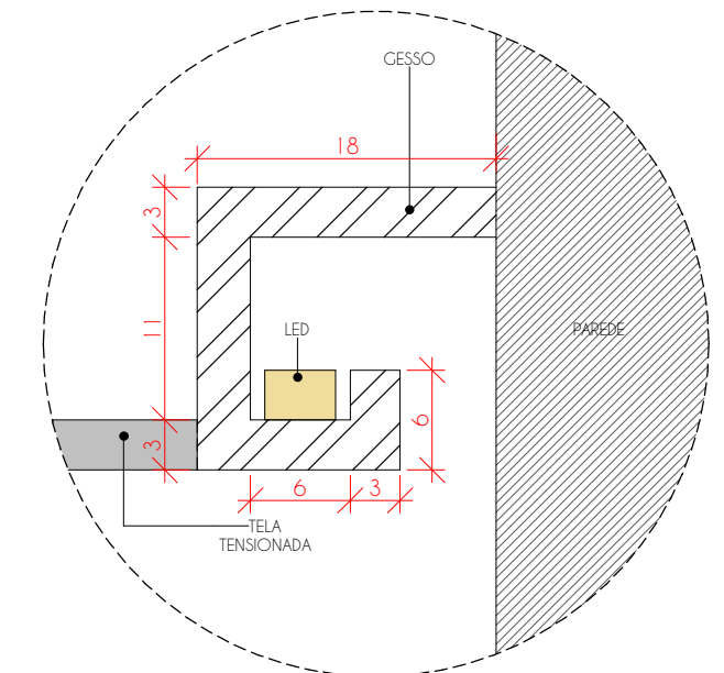
DET. TELA TENSIONADA ESCALA 1 : 5
