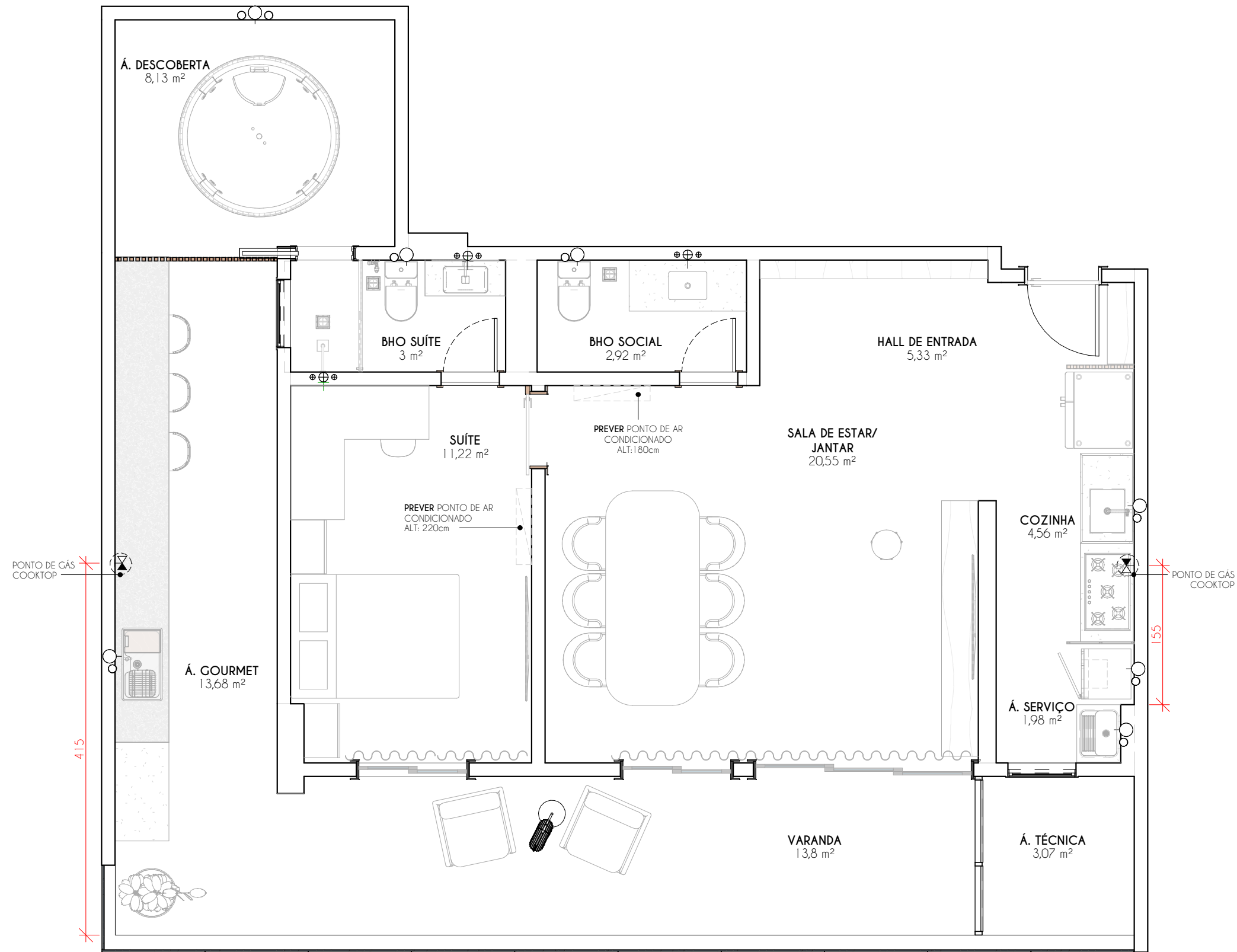
PLANTA BAIXA- PONTOS HIDRÁULICOS
