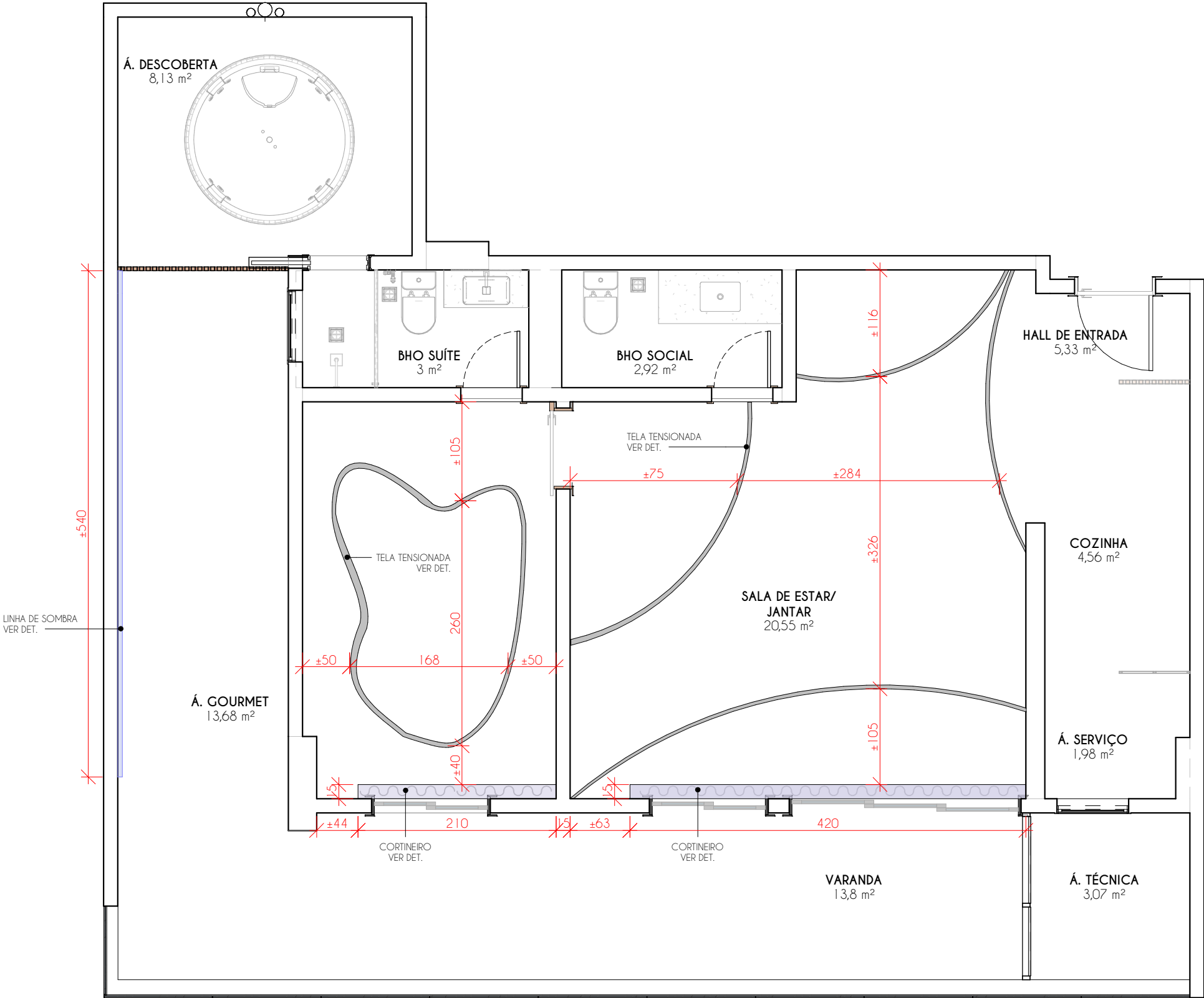
PLANTA BAIXA- GESSO ESCALA 1 : 50
