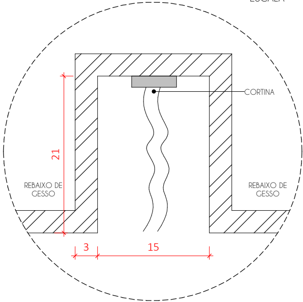
DET. CORTINEIRO ESCALA 1 : 5
