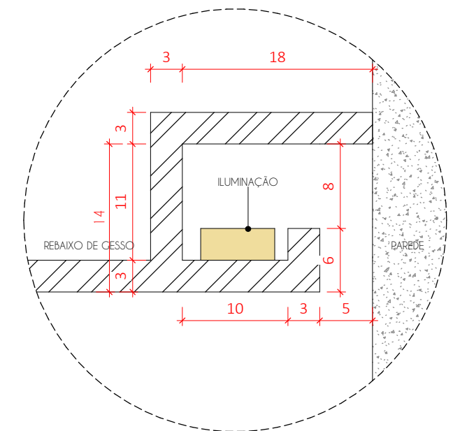
DET. LINHA DE SOMBRA ESCALA 1 : 5
