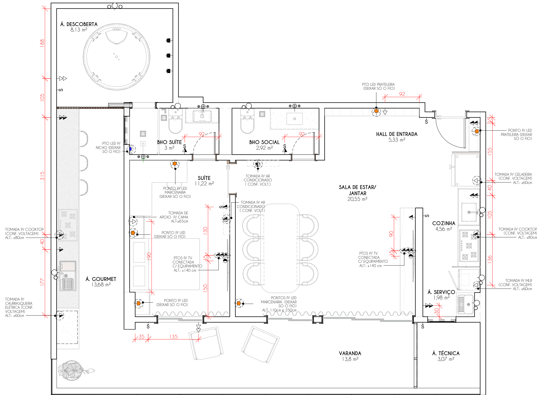
PLANTA BAIXA- PONTOS ELÉTRICOS ESCALA 1 : 50
