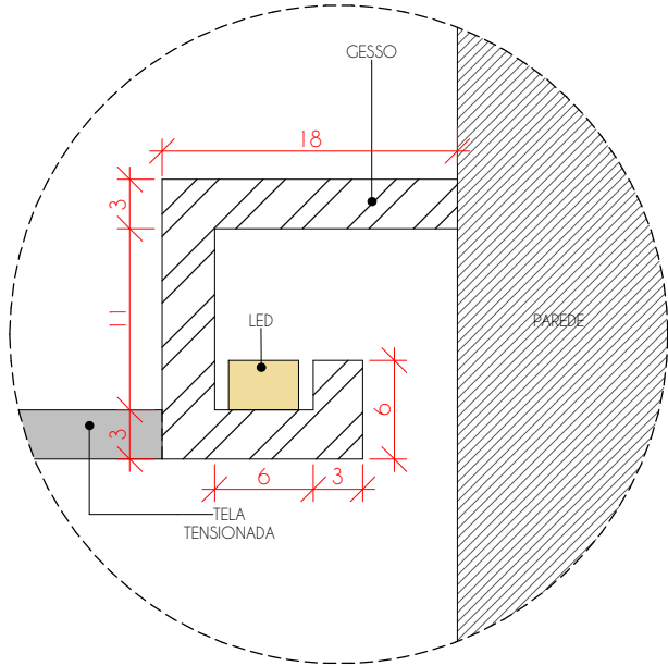
DET. TELA TENSIONADA ESCALA 1 : 5
